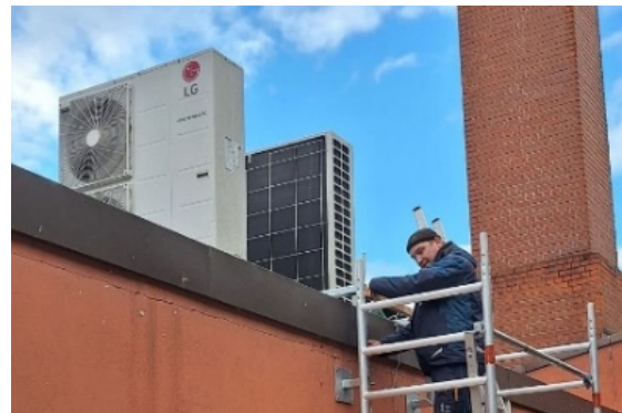
Montage von Wärmepumpen auf dem Wirtschaftshof in Wörlitz © KsDW, Robert Hartmann
